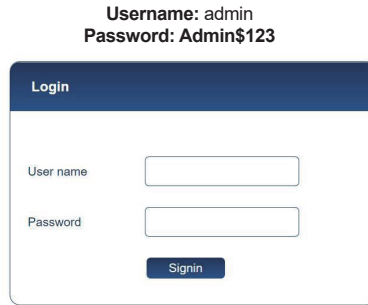
Figure 4. WebUI login
