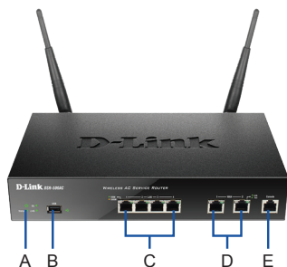
圖片1. DSR-500AC/1000AC 面板
