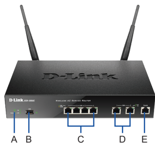
Рис.1 Передняя панель DSR-500AC
