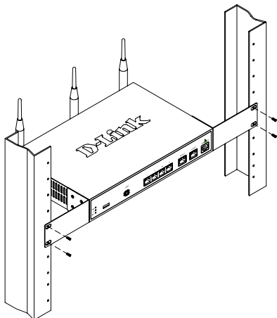
Рис.4 Установка маршрутизатора в стандартную стойку
