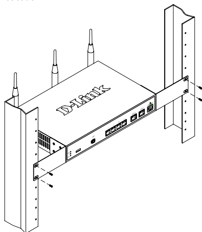
Figura 4. Instalação do Wireless AC Services Router num bastidor de equipamento de tamanho padrão
