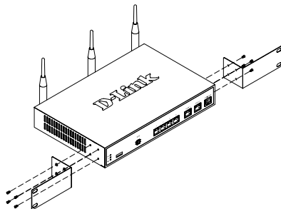
Gambar 3. Memasang Braket Pemasangan Rak
