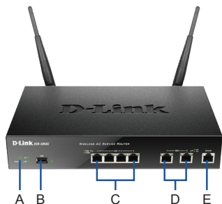
Мал.1 Передня панель DSR-500AC/1000AC
