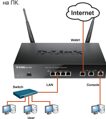
Малюнок 3. Приклад підключення основних кабелів
