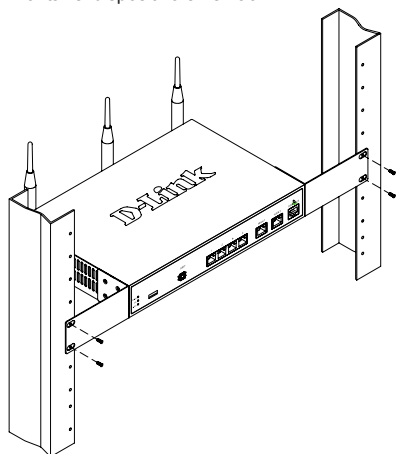
Figura 4. Instale el Router de Servicios Wireless AC Gigabit en un rack de equipos tamaño estándar
