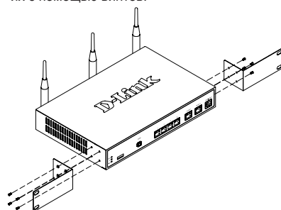
Рис.3 Прикрепление скоб для установки в стойку
