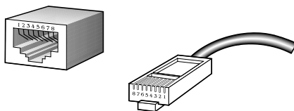
Connecteur standard RJ-45 femelle/mâle
