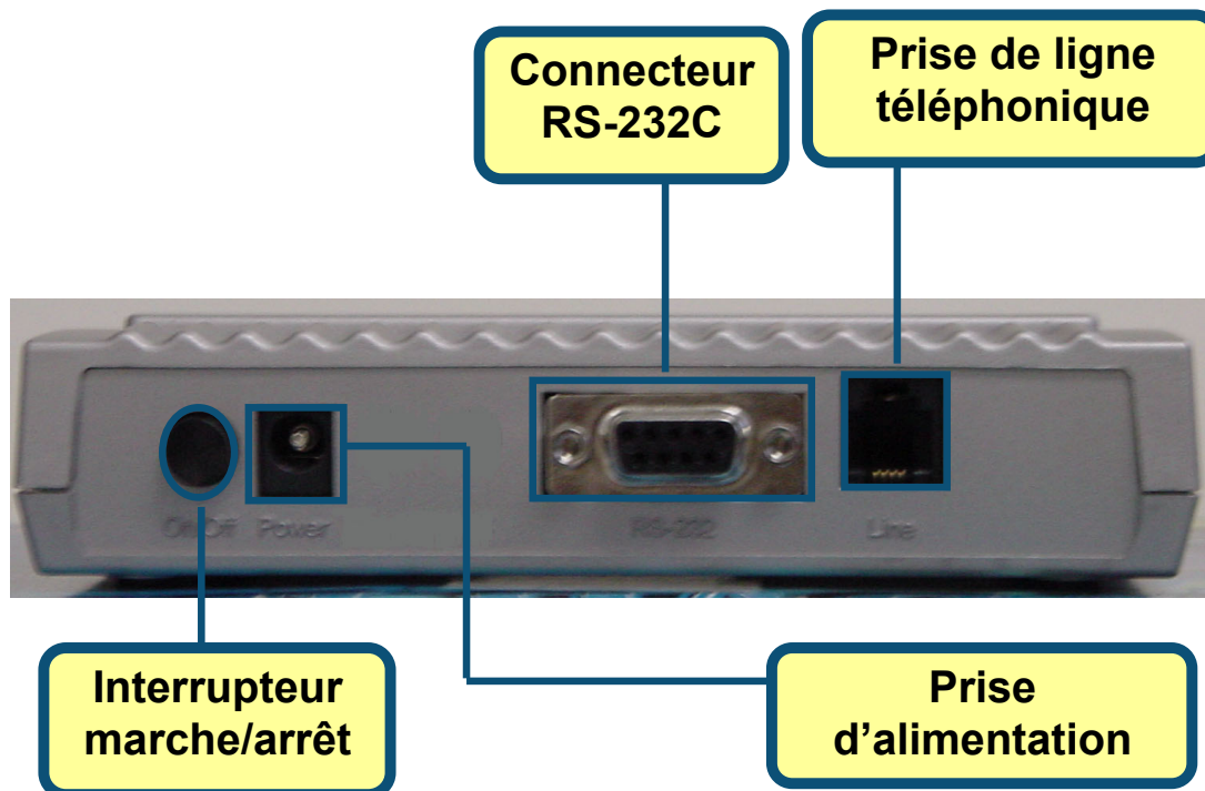
Schéma d'installation du modem externe
