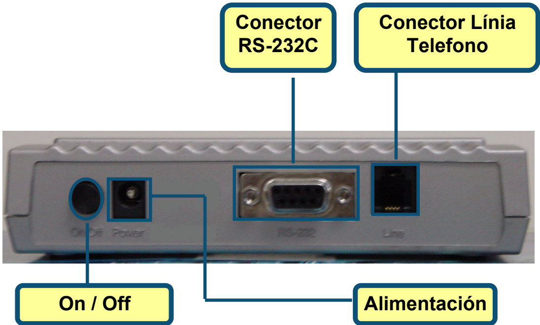
Diagrama Módem Externo
