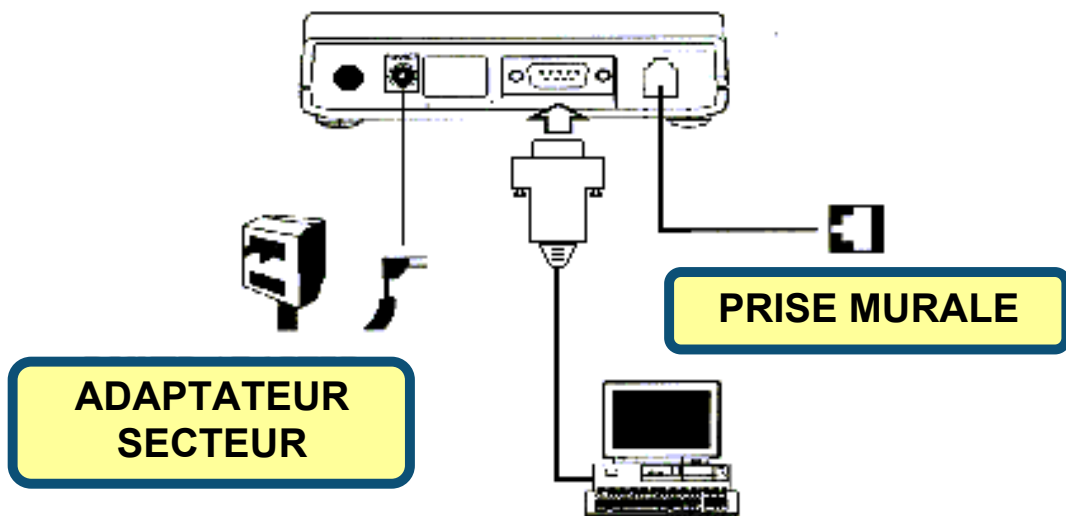
Schéma d'installation du modem externe
